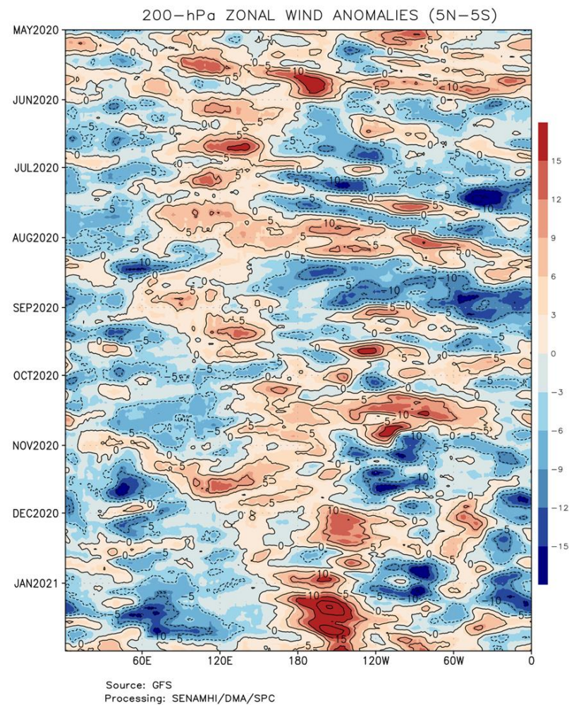
Figura 5. Anomalías de vientos zonales a 850 hPa (a) y 200 hPa (b) entre los 5°S y 5°N en la franja ecuatorial de mayo 2020 a enero 2021. Procesamiento: SENAMHI.
