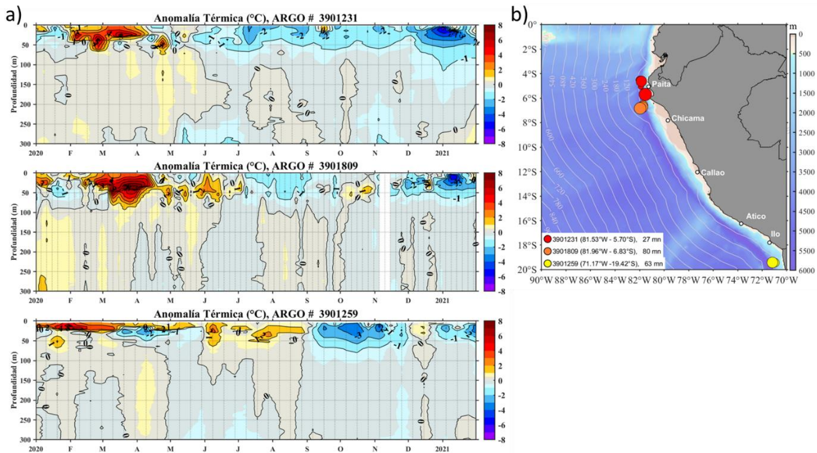
Figura 17. Evolución de la anomalía de la temperatura del agua de mar en flotadores ARGO cerca a la costa (a); y ubicación de las últimas posiciones y coordenadas geográficas para el mes de enero donde brindaron información los flotadores ARGO (b). Fuente: ARGO, climatología: 1981-2010. Procesamiento: AFIOQ/DGIOCC/IMARPE.
