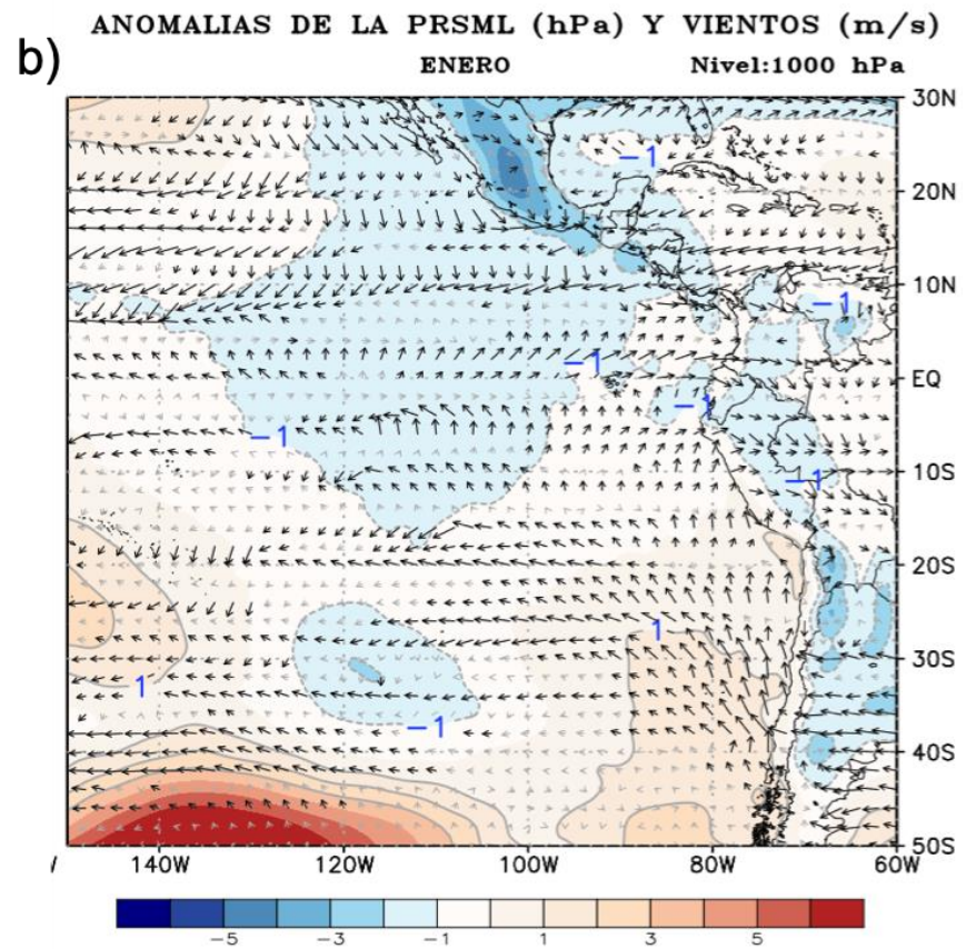
Figura 8. Promedio mensual (izquierda) y anomalías (derecha) de la presión reducida a nivel del mar (PRSML, colores) y vientos (flechas) para enero 2021. Procesamiento: SENAMHI.
