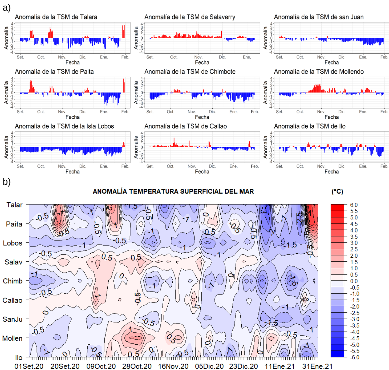
Figura 12. Anomalia de TSM diaria a lo largo de la costa peruana durante los últimos 5 meses, a) serie y b) hövmoller. Actualizado al 31 de enero 2021. Climatología: 1981-2010. Fuente: DIHIDRONAV.
