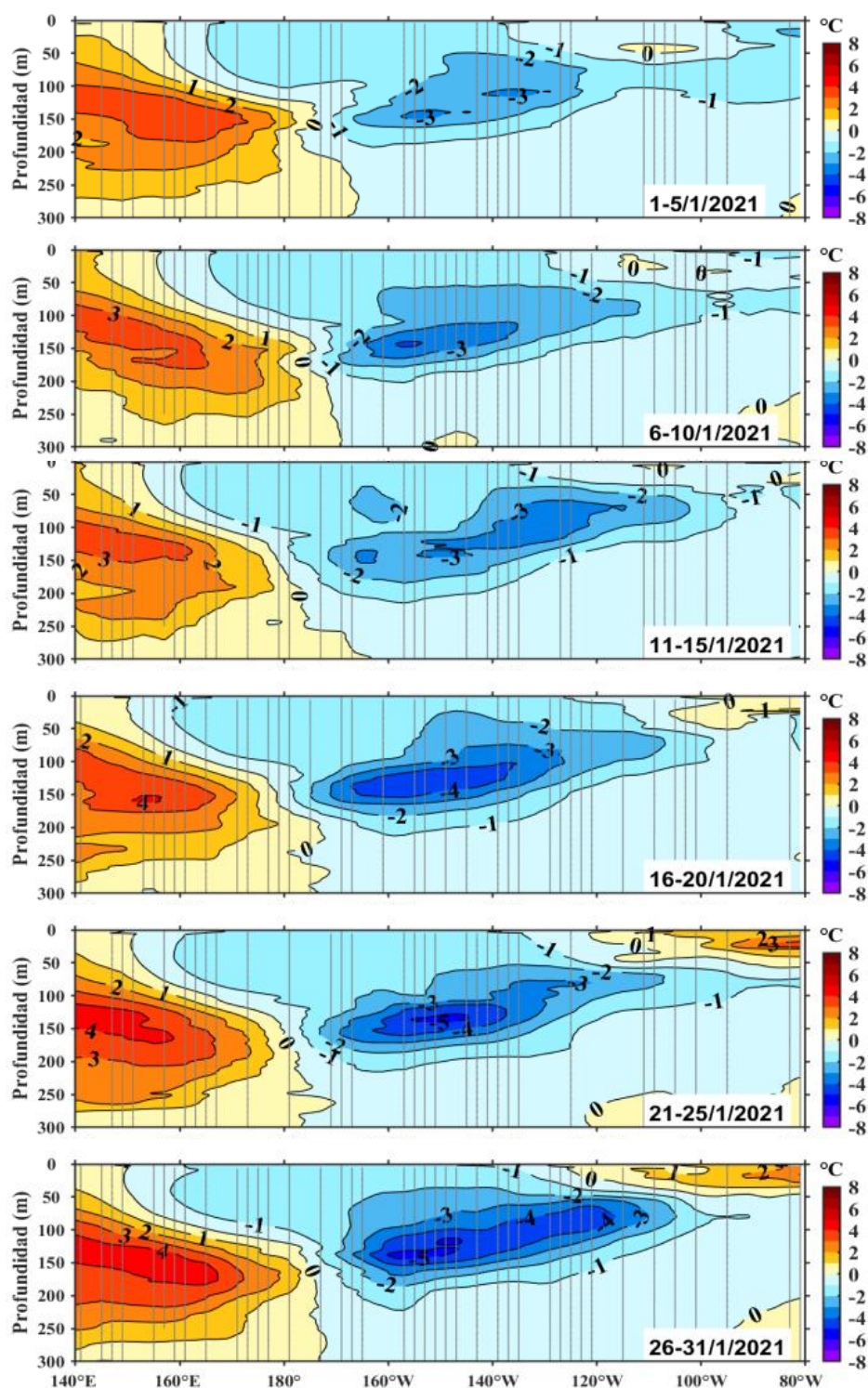
Figura 3. Anomalías de temperatura ( ^{\circ}\text{C} ) en la capa superior (0-500 m) del Pacífico Ecuatorial ( 2^{\circ}\text{S} - 2^{\circ}\text{N} ), en promedios de cinco días durante enero de 2021 (las fechas indican el último día, los contornos están separados a 1^{\circ}\text{C} ). Periodo base: 1981-2010. Fuente: ARGO – TAO/TRITON, Adaptado: PMEL/NOAA.
