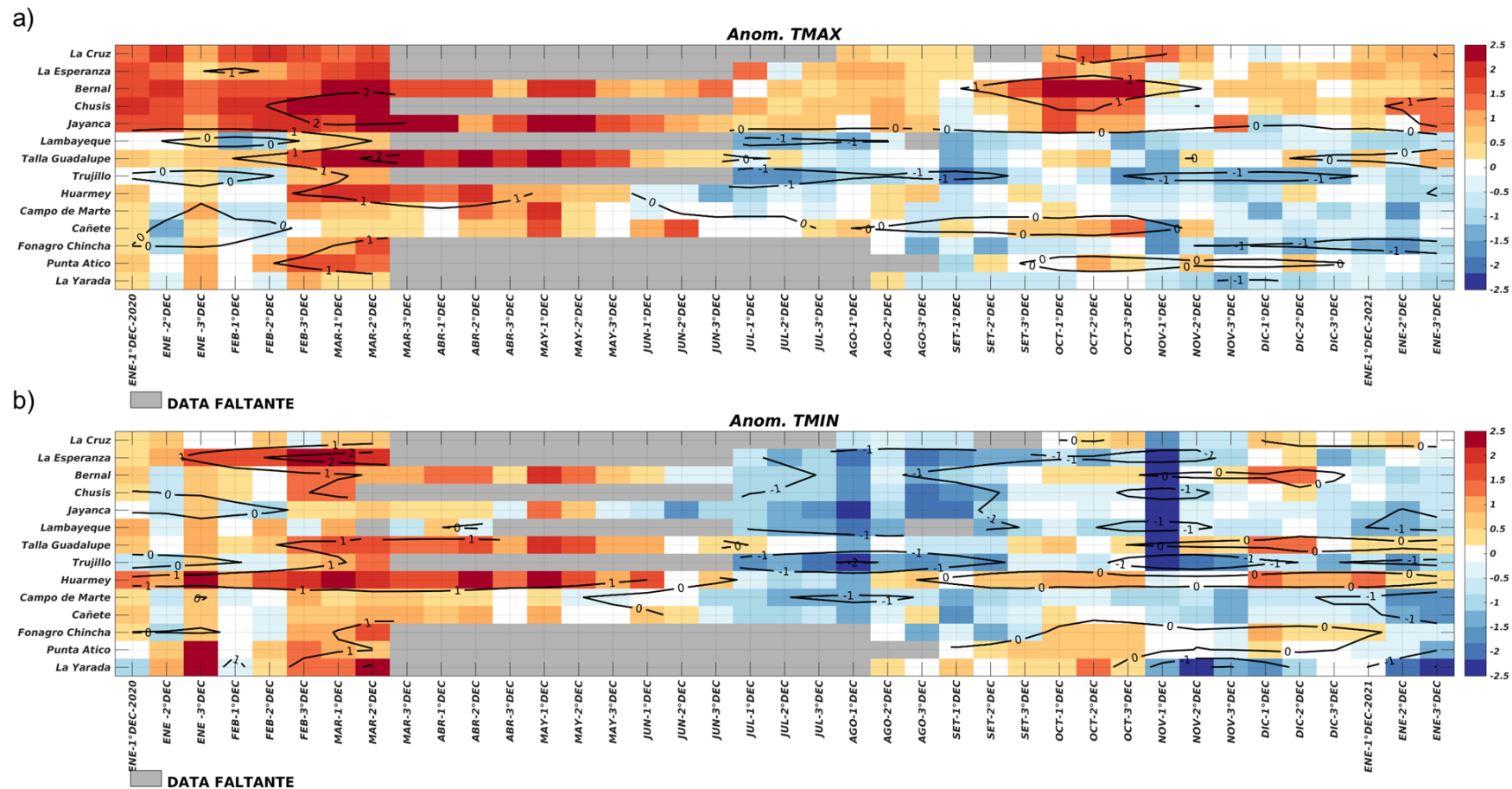
Figura 10. Temperaturas del aire máxima (a) y mínima (b) en las estaciones costeras de SENAMHI entre enero 2020 hasta enero 2021 Fuente: SENAMHI.
