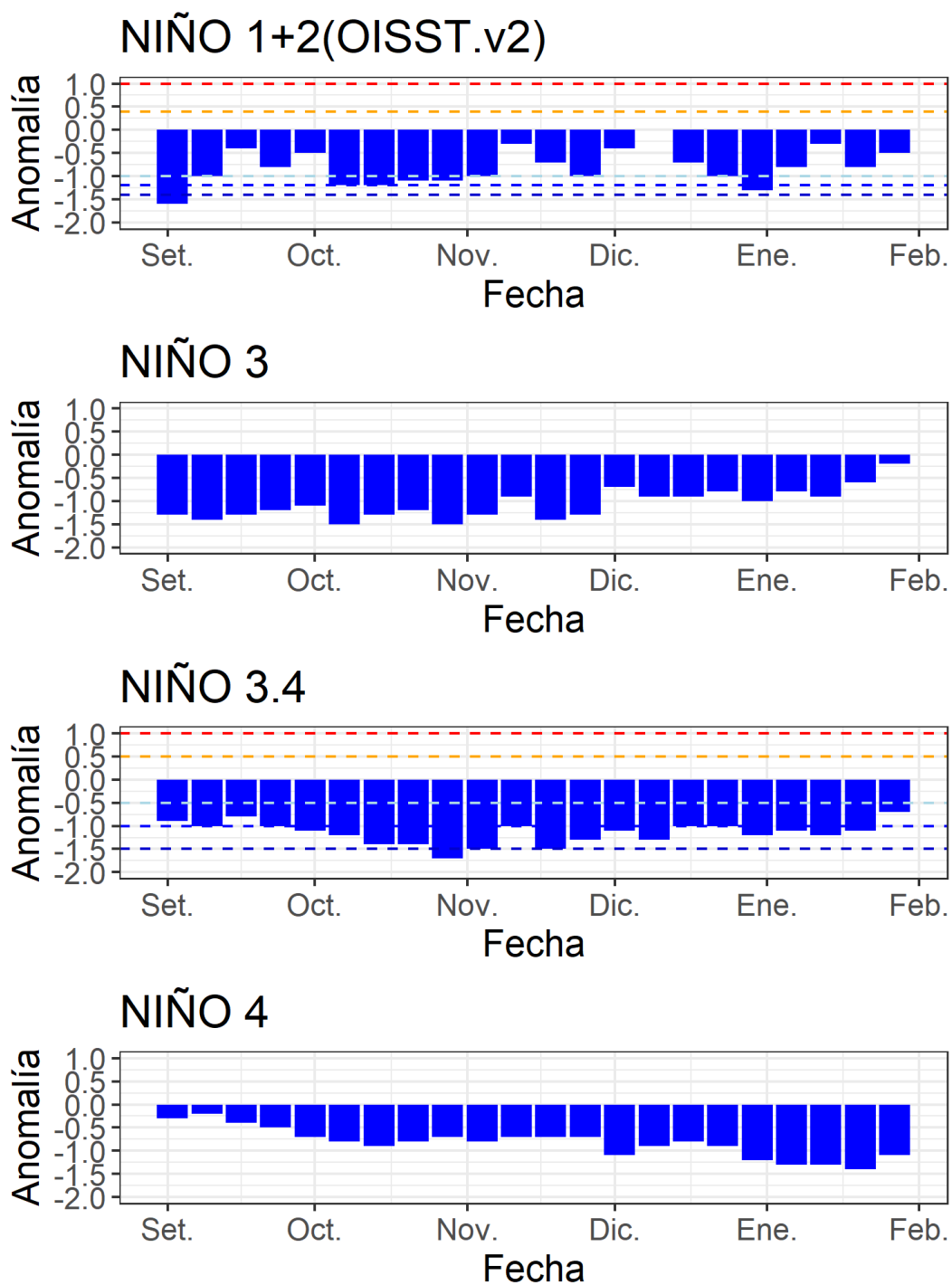
Figura 2. Series de tiempo de las anomalías semanales de la TSM (°C) en las regiones Niño, de setiembre 2020 a enero del 2021. Fuente: AVHRR NCEP/NOAA; procesamiento: DIHIDRONAV.
