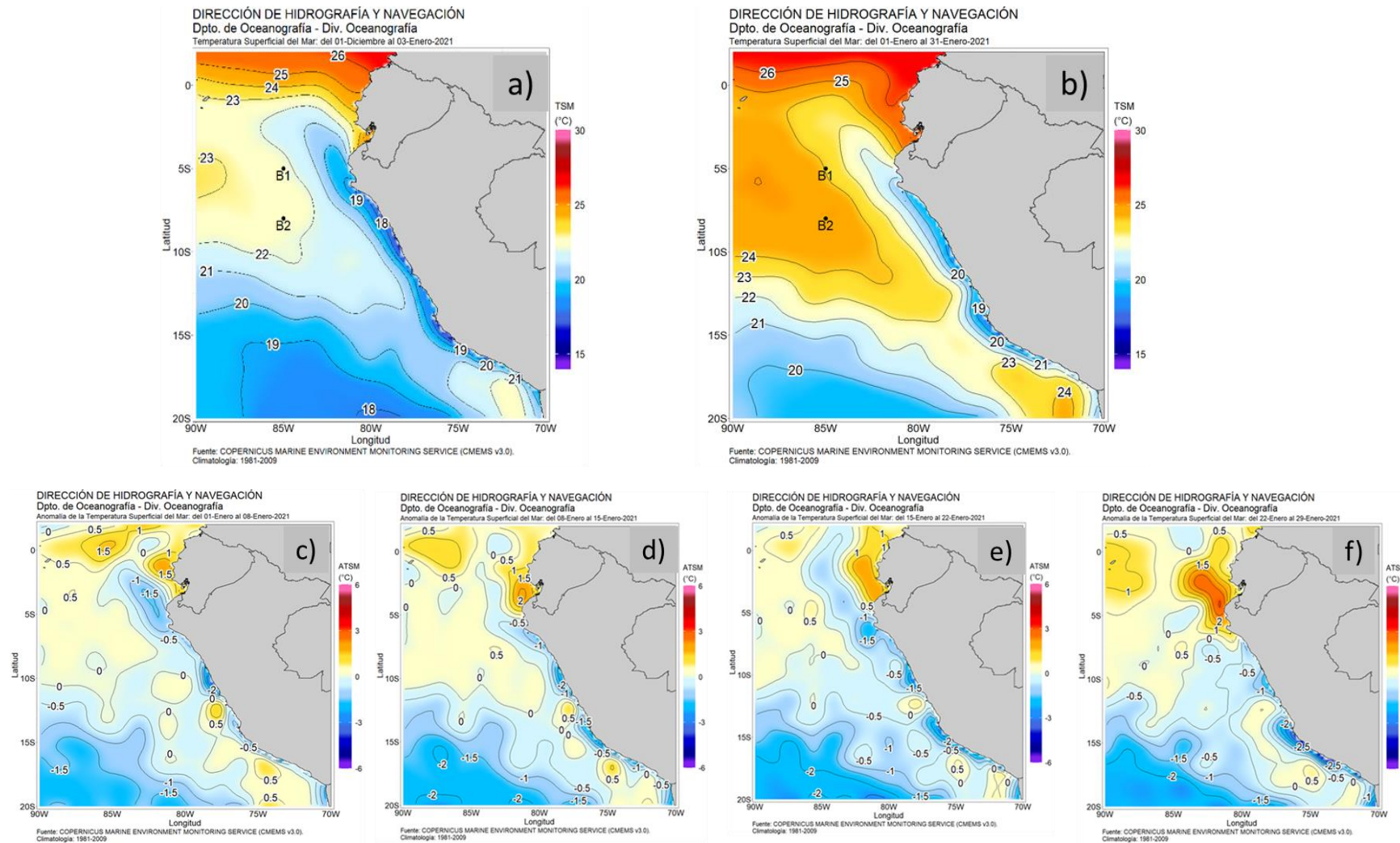
Figura 13. Mapa de distribución espacial de la TSM (°C) mensual durante diciembre 2020 (a) y enero 2021 (b), y de las anomalías de la TSM (°C) (c-f) semanal durante enero 2021 en el océano Pacífico tropical oriental. Fuente: CMEMS v3.0. Procesamiento: DIHIDRONAV.
