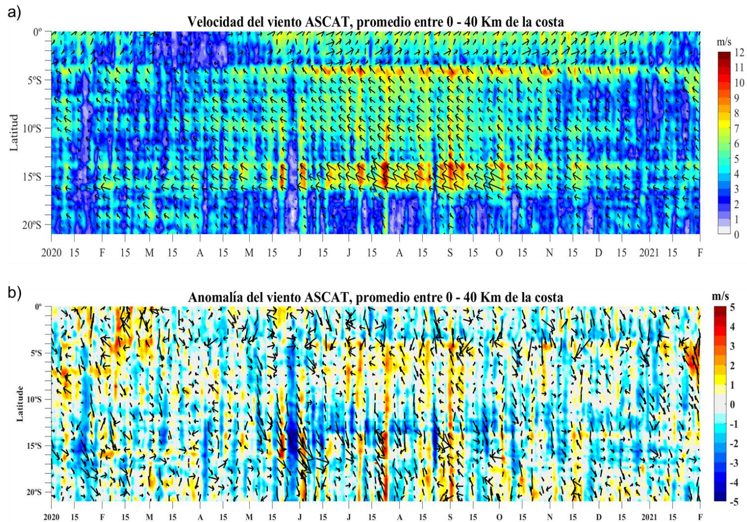
Figura 9. a) Velocidad del viento ( \text{m s}^{-1} ), y b) anomalía del viento ( \text{m s}^{-1} ), desde los 0° hasta 20°S en el periodo durante los últimos 12 meses. Los vectores representan la dirección del viento y anomalía de la dirección del viento, respectivamente. Actualizado al 31 de enero 2021. Datos: ASCAT. Procesamiento: IMARPE.
