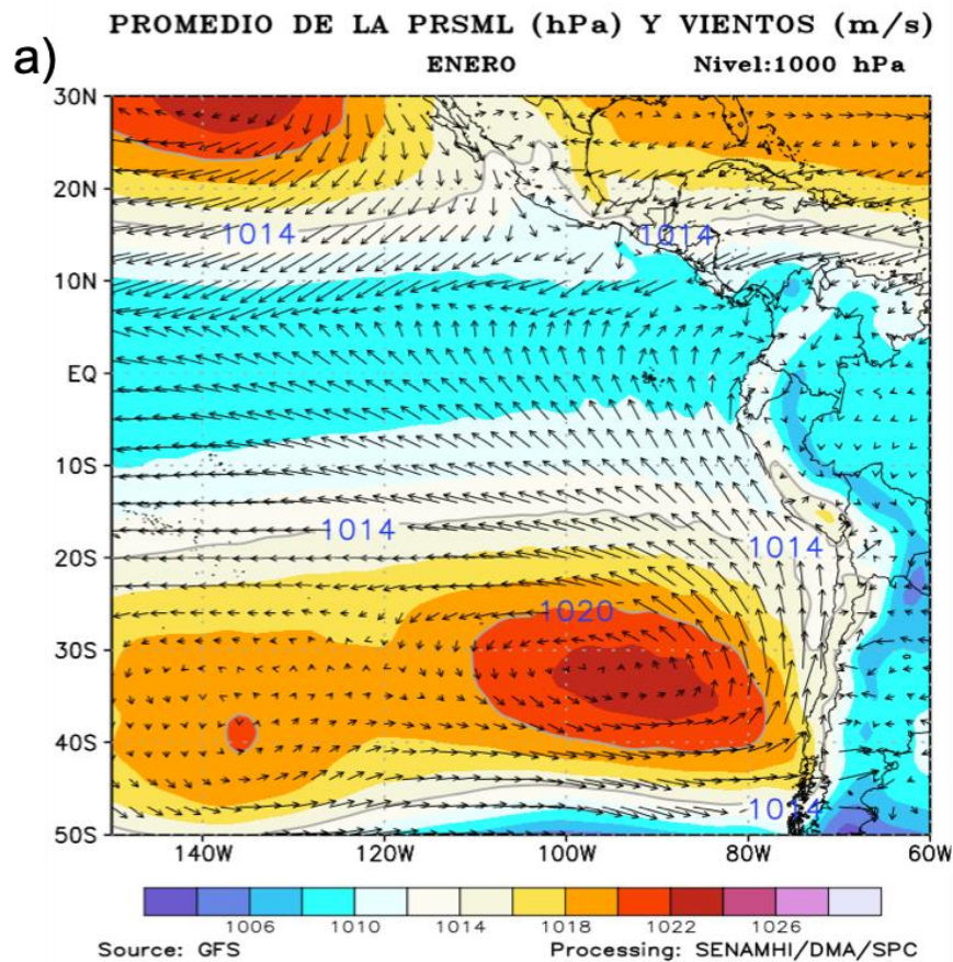
Figura 8. Promedio mensual (izquierda) y anomalías (derecha) de la presión reducida a nivel del mar (PRSML, colores) y vientos (flechas) para enero 2021. Procesamiento: SENAMHI.
