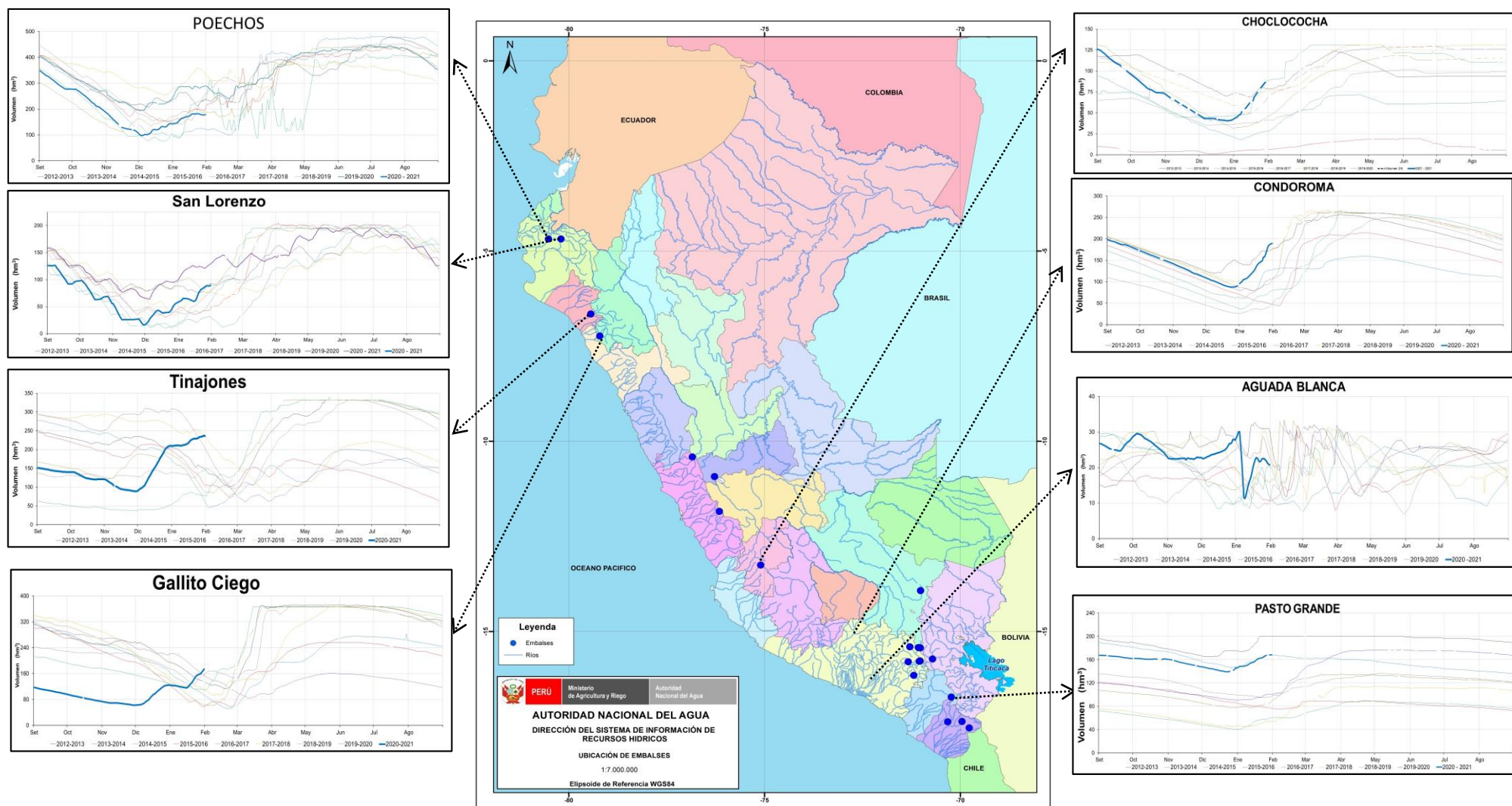
Figura 25. Volúmenes de almacenamiento ( \text{hm}^3 ) de los principales Embalses del norte (izquierda), centro (derecha) y sur (derecha) del Perú, actualizado hasta 31 de enero 2021. Las líneas azules indican volúmenes de almacenamiento del año hidrológico 2020-2021, líneas rojas, amarillo, verdes y negro: corresponden a años hidrológicos 2019 – 2020, 2018-2019, 2017-2018, 2016-2017, 2014-2015. Fuente: PE Chira-Piura, JU's San Lorenzo, Chancay Lambayeque, AUTODEMA, GORE PERPG, EGESUR. Procesamiento: ANA.
