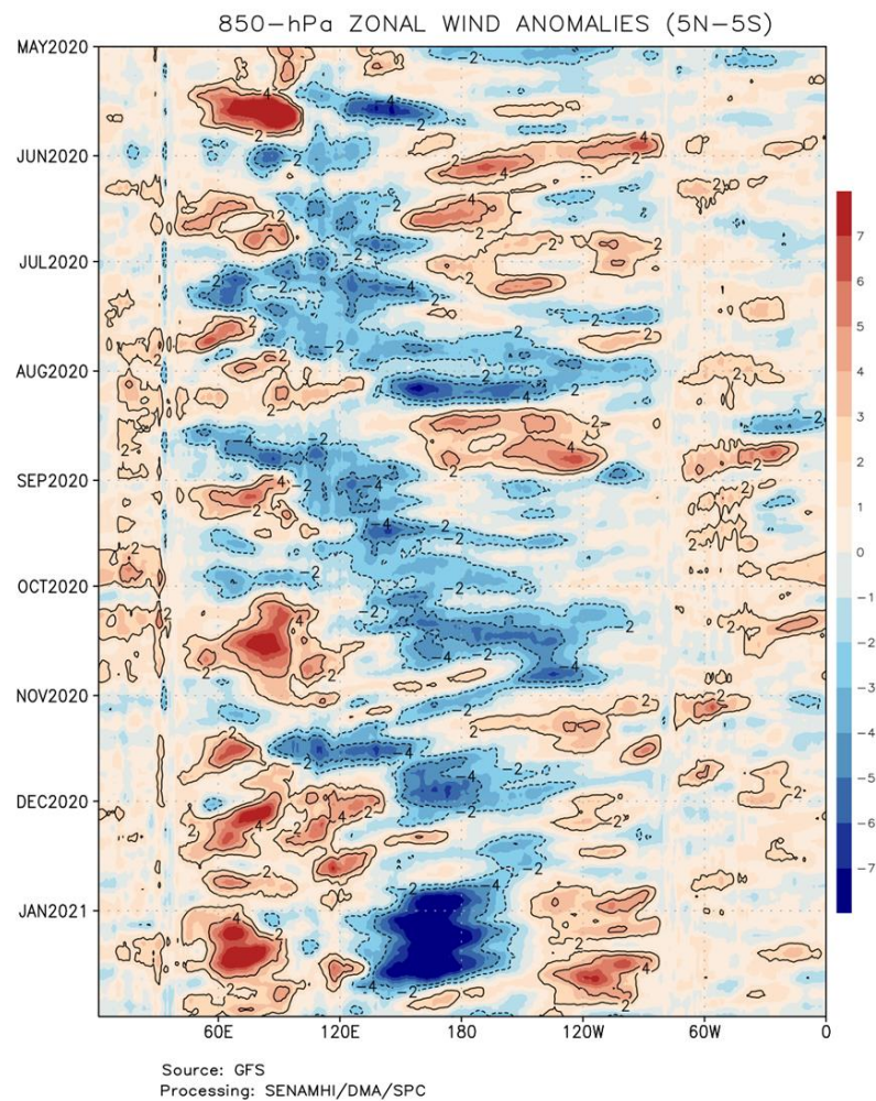
Figura 5. Anomalías de vientos zonales a 850 hPa (a) y 200 hPa (b) entre los 5°S y 5°N en la franja ecuatorial de mayo 2020 a enero 2021. Procesamiento: SENAMHI.
