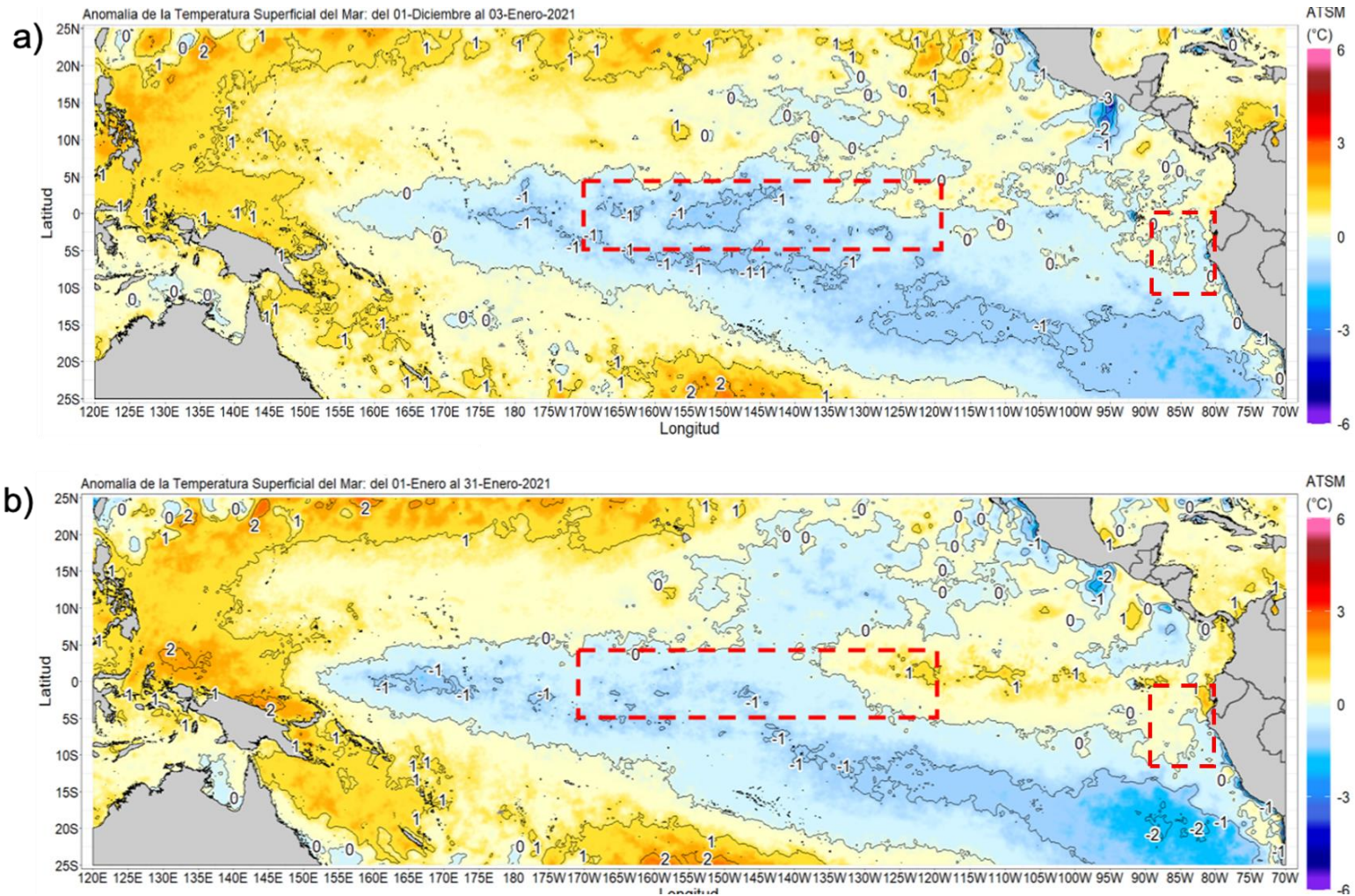
Figura 1. Promedio mensual de las anomalías de TSM en el Pacífico central durante diciembre 2020 (a) y enero 2021 (b). Las regiones El Niño 3.4 y El Niño 1+2 están delimitadas con los recuadros rojos. Fuente: CMEMS v.3.0, Procesamiento: DIHIDRONAV.
