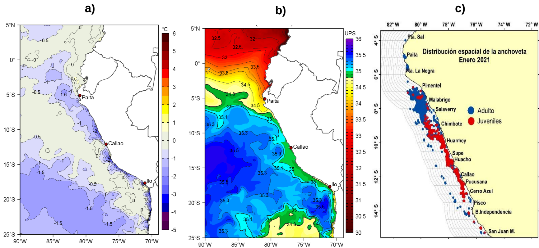
Figura 19. a) Temperatura superficial del mar - TSM (°C), b) Salinidad superficial del mar - SSM (ups) y c) Distribución de la anchoveta durante enero 2021 en la región norte – centro. Fuente: IMARPE.
