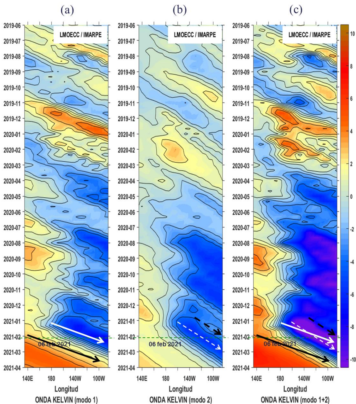
Figura 27. Diagrama Hovmöller de longitud-tiempo de las ondas Kelvin oceánicas en el Pacífico ecuatorial: (a) Modo 1, (b) Modo 2, (c) Modo 1+ Modo 2. El modelo fue forzado con información de NCEP. La línea discontinua horizontal de color verde indica el inicio del pronóstico sin el forzante de viento; fecha inicial del pronóstico: 06 de febrero 2021. Fuente: IMARPE.
