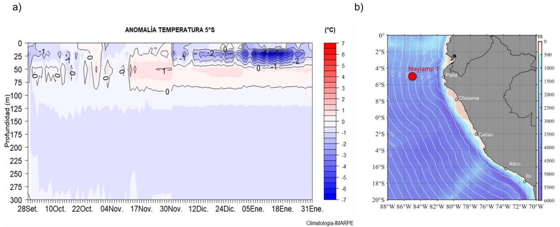
Figura 16. Evolución de la anomalía de la temperatura del agua de mar en la a) en la boya Naylamp 1 y b) su ubicación (85° W – 5° S). Procesamiento: DIHIDRONAV.
