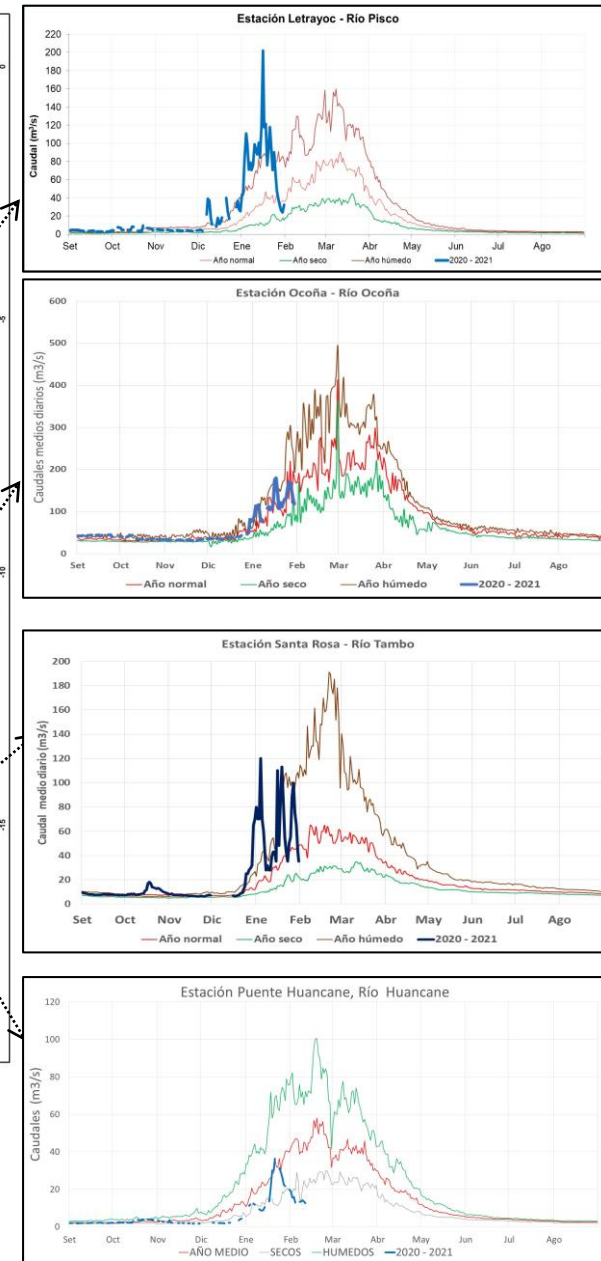
Figura 24. Caudales diarios ( m^3 s^{-1} ) de los principales ríos del norte (izquierda), centro (centro) y sur (derecha) del Perú, actualizado hasta 31 de enero 2021. Las líneas azules indican caudales del año hidrológico 2020-2021, rojas: caudales normales; Fuente: SENAMHI, Proyectos Especiales y Juntas de Usuarios. Procesamiento: ANA.
