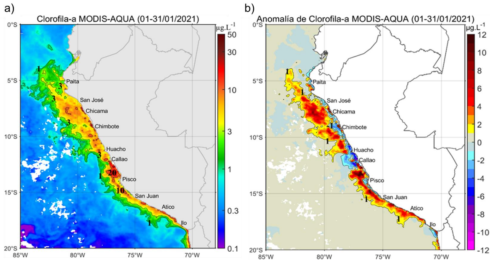
Figura 18. Mapa de la concentración de clorofila-a superficial satelital (a) y su anomalía (b y d) durante enero de 2021, proveniente de MODIS-AQUA ( \mu\text{g L}^{-1} ). En (c), se muestra la serie de tiempo de las concentraciones de clorofila-a satelital (barras negras) y su climatología (línea verde) proveniente de SeaWiFS-MODIS ( \mu\text{g L}^{-1} ) entre 4°S-16°S y dentro de los 100 km de la costa. Fuente: IMARPE.
