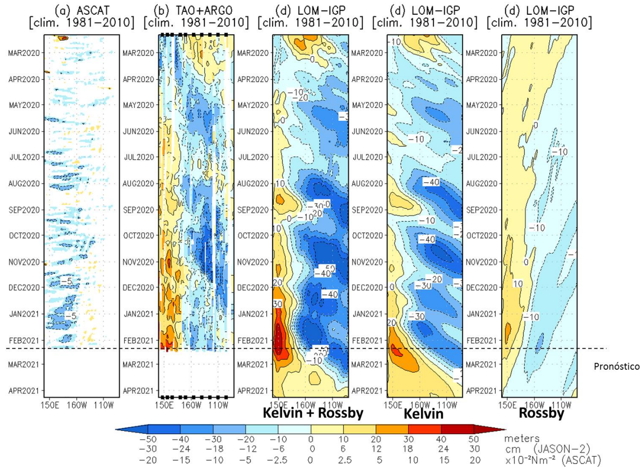
Figura 26. Diagrama longitud-tiempo de las anomalías de esfuerzo de viento zonal ecuatorial basado en datos de ASCAT (a), anomalía de la profundidad de la isoterma de 20 °C con datos de TAO y los derivadores de Argo (b), diagrama de la onda de Kelvin y Rossby (c), diagrama de la onda de Kelvin (d) y finalmente diagrama de la onda de Rossby (e), calculado con el Modelo oceánico lineal (LOM-IGP), forzando por ASCAT y tau=0 para el pronóstico. La línea roja discontinua representa el inicio del pronóstico Procesamiento: IGP.
