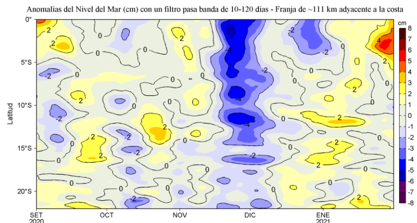
Figura 11. Anomalías del NMM, actualizado al 31 de enero del 2021: a) Diagrama Hovmöller durante el último semestre en estaciones costeras de la DIHIDRONAV; b) Diagrama Hovmöller de las anomalías del nivel del mar diario (cm) sin filtro; y c) con filtro pasa banda de 10 a 120 días, para la franja de 60 millas náuticas adyacente al litoral peruano. Fuente: CMEMS v3.0; Climatología: 1993-2012. Procesamiento: LHFM/AFIOF/DGIOCC/IMARPE.
