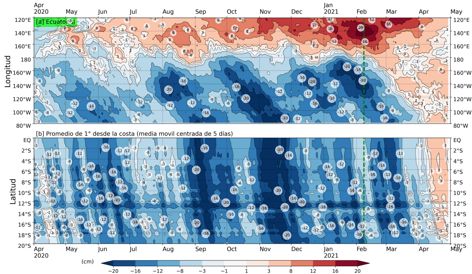
Figura 28. Anomalia del nivel del mar (en cm) para la sumatoria de los modos (modo 1, 2 y 3) simulado a partir del Modelo Oceánico Multimodal (MOMM-IGP; Urbina y Mosquera, 2020) en la franja ecuatorial (superior) y costera (inferior). La línea verde representa el inicio del pronóstico. El modelo fue forzado con la fuente de datos de viento denominada BLENDED (Bentamy et al., 2016). Fuente: IGP.
